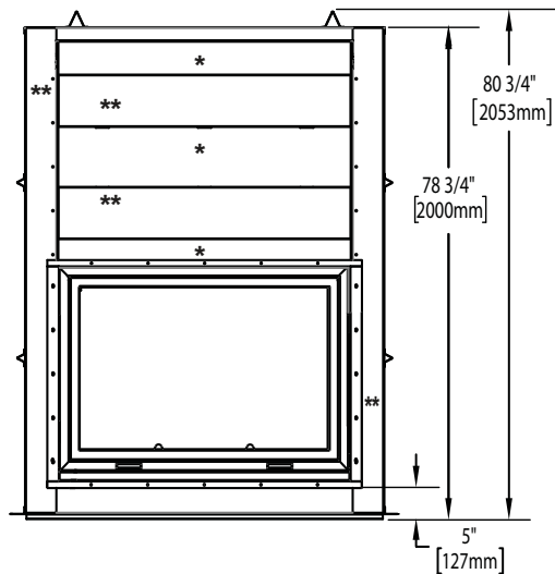
NZ8000 ILLUSTRATED * NE VIS PAS DANS CE RÉGION ** NE VIS PAS DE 1/2" PLUS CE RÉGION
