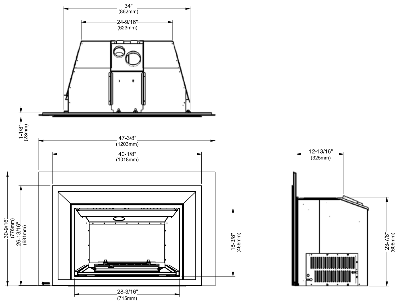
Dimensions with Vignette Faceplate
