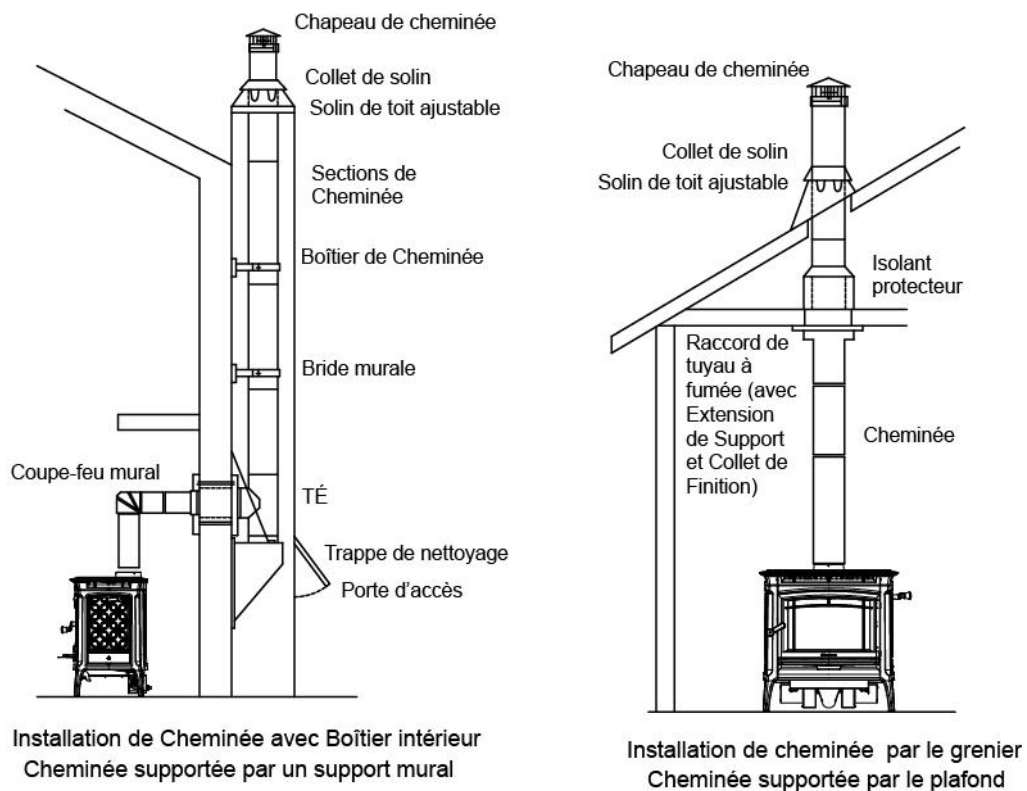
Figure 7 – Configurations de Cheminée
