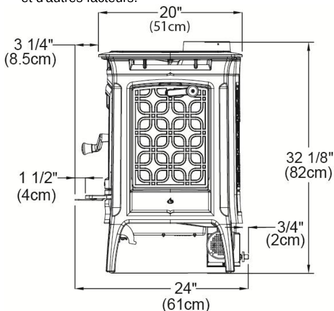
Figure 1 – Dimensions du Manchester
