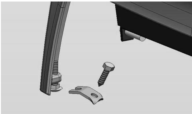
Figure 9 - Fixation du poêle dans le plancher
