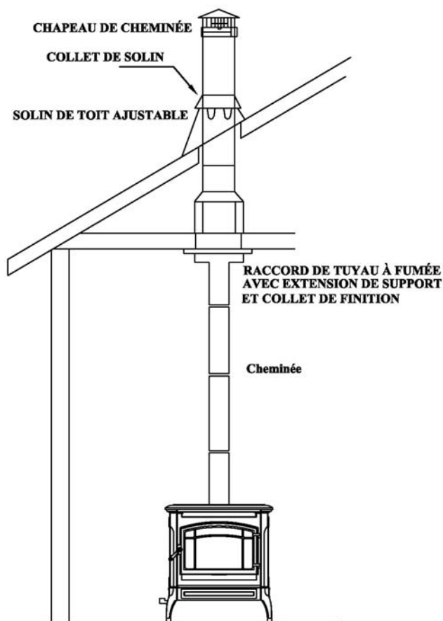
Installation Typique de Maison Mobile. Cheminée supportée par le Plafond.
