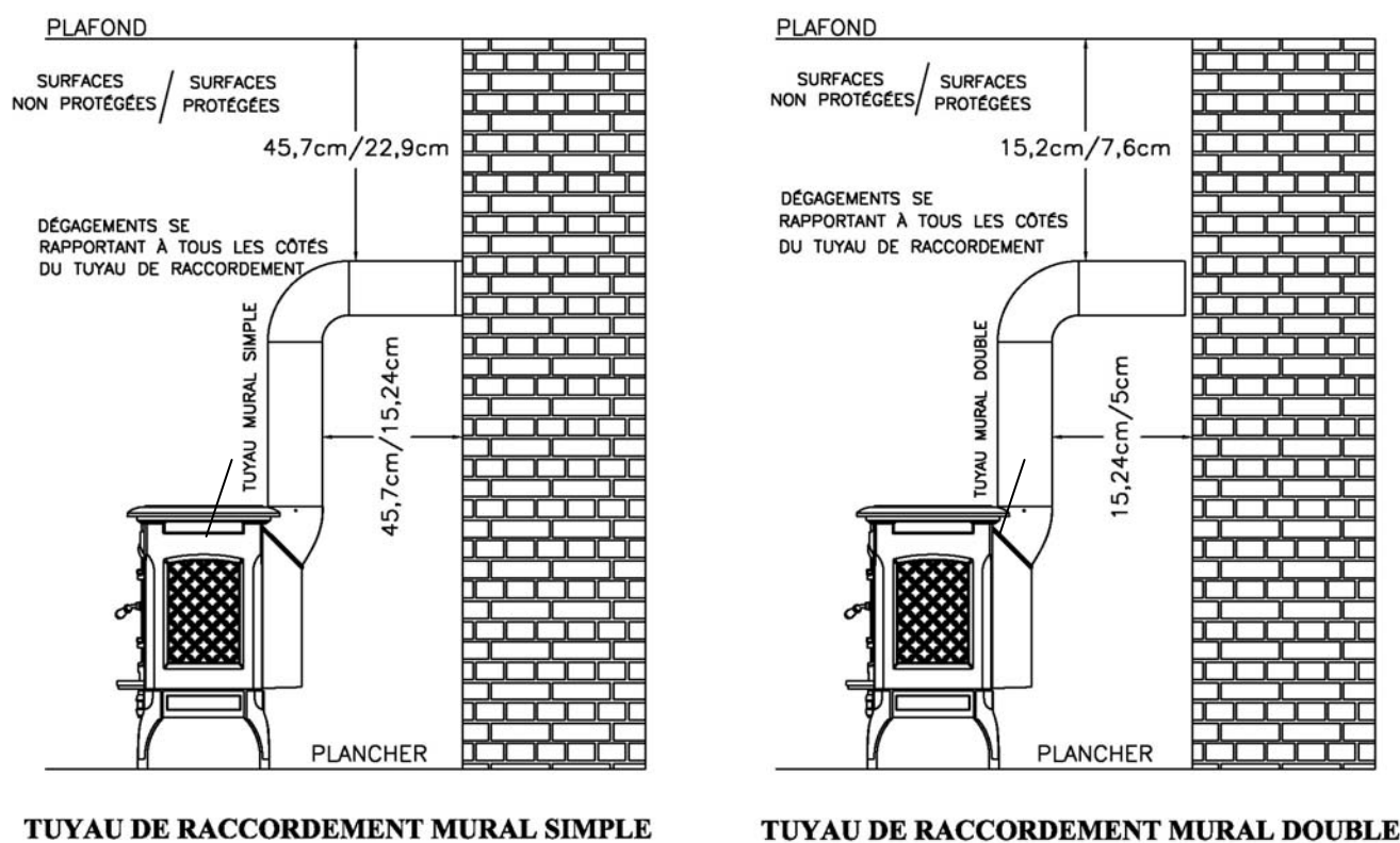
Figure 7 - Dégradement des Tuyaux de Raccordement
