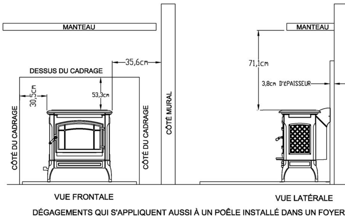
Figure 6 – Dégradements d'Installation du Poêle
