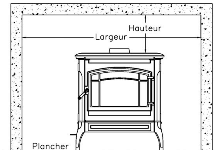
Figure 5 – Dégagements d'une Installation en Alcôve
