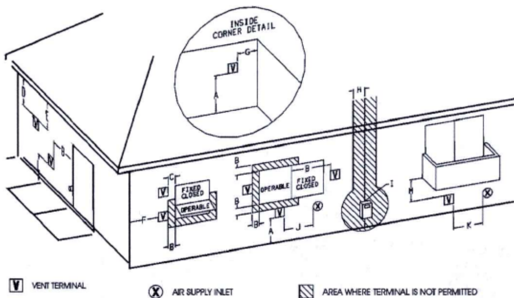
Figure 11: Emplacement acceptable de la terminaison
