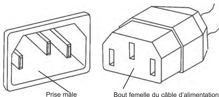
Branchement de l'alimentation principale
