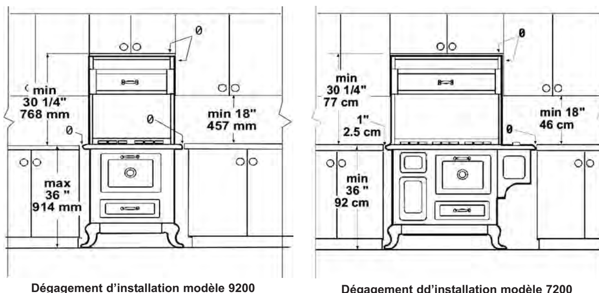
Figure 2 Dégagements d'installation
