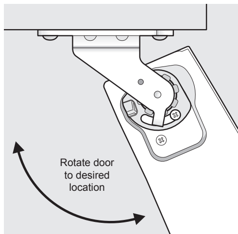
Adjusting door
