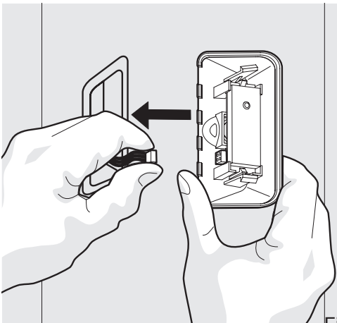
Retrait du faisceau électrique de la DEL Figure 55
