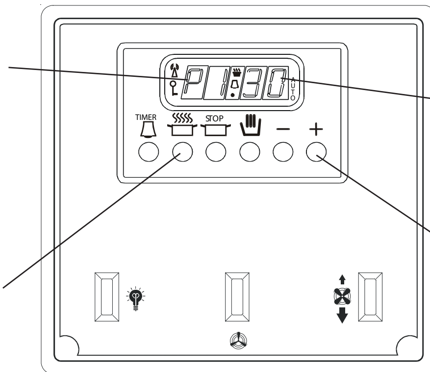
Figure A - Disposition du tableau de commande
