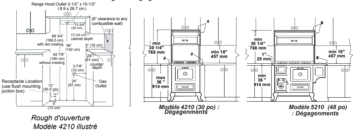
Fig 3 Dégagements d'installation
