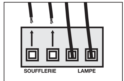
SOUFFLERIE/LAMPE BORNIER (VUE DE SUPÉRIEURE)
