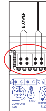
SOUFFLERIE/ LAMPE BORNIER
