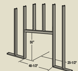
LBR-3824 FRAMING
