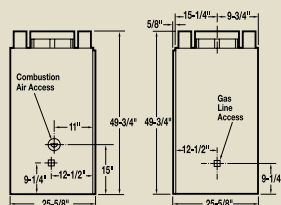
LBR-3824 FRAMING
