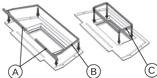
Replace gaskets A, B and C. * Remplacez les joints A, B et C. *
