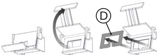
Open dilution door & remove gasket. Ouvrez la porte de dilution et retirez le joint.
