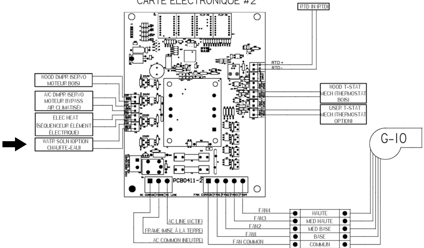
CARTE ÉLECTRONIQUE #2
