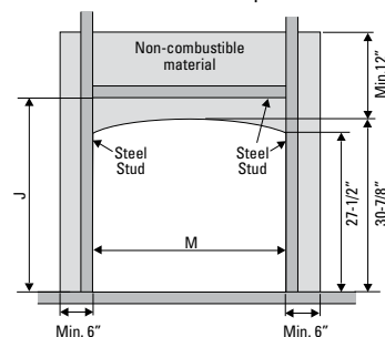
FRONT FRAMING DIMENSIONS*** P36 /P36E/P36D Tripoli
