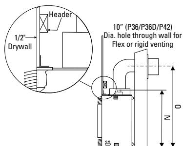
MINIMUM TERMINATION CENTER LINE P36/P36E/P36D/P42
