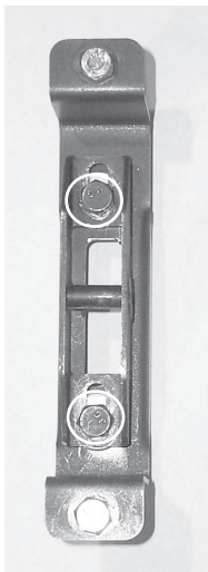
L a t c h A s s e m b l y r e - a s s e m b l e d w i t h s p a c e r s r e m o v e d .
