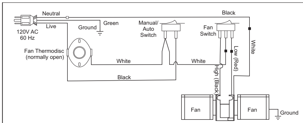
Fan Wiring Diagram
