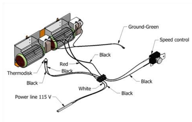
Figure 22 – Fan Wiring
