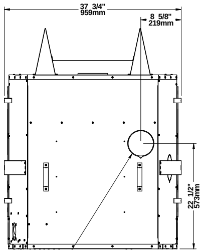
ENSEMBLE AIR PULSÉ 6\"/>
