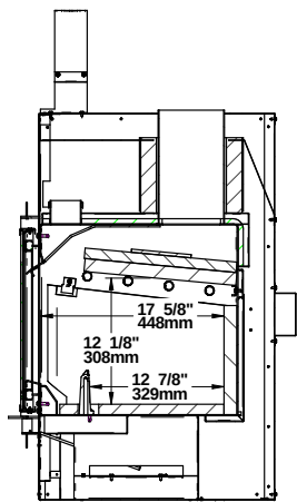
SECTION A-A
