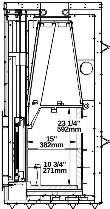
SECTION D-D
