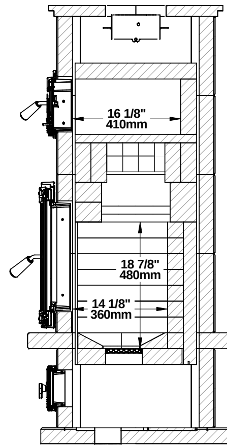
SECTION A-A
