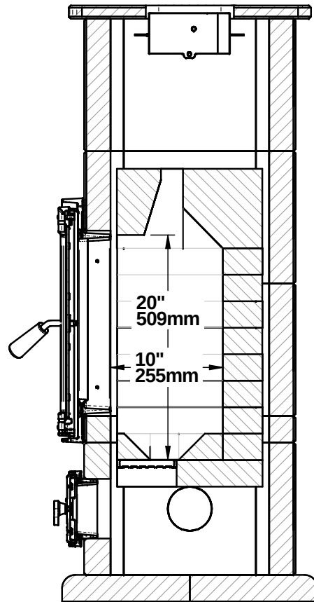
SECTION A-A
