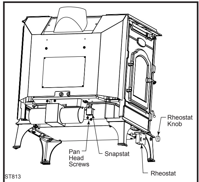
Fig. 23 Fan installation.
