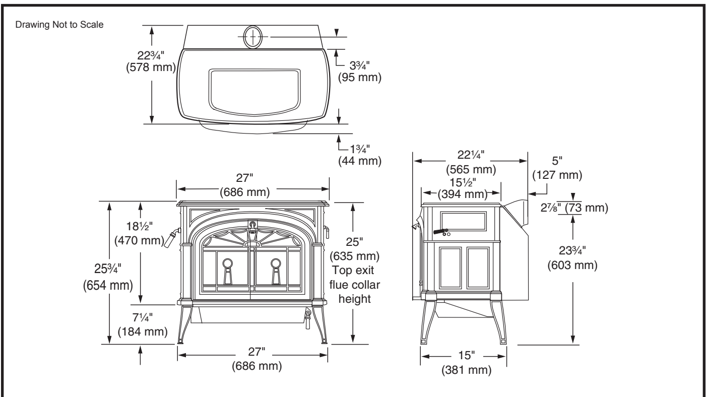
Fig. 1 Encore 2040 dimensions.
