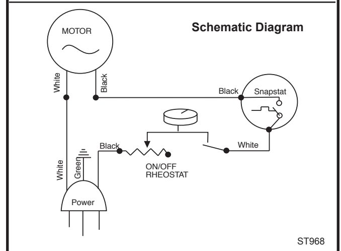
Fig. 85 Fan circuit.
