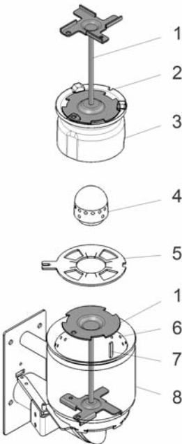
Fig. 121 BioWIN 150
