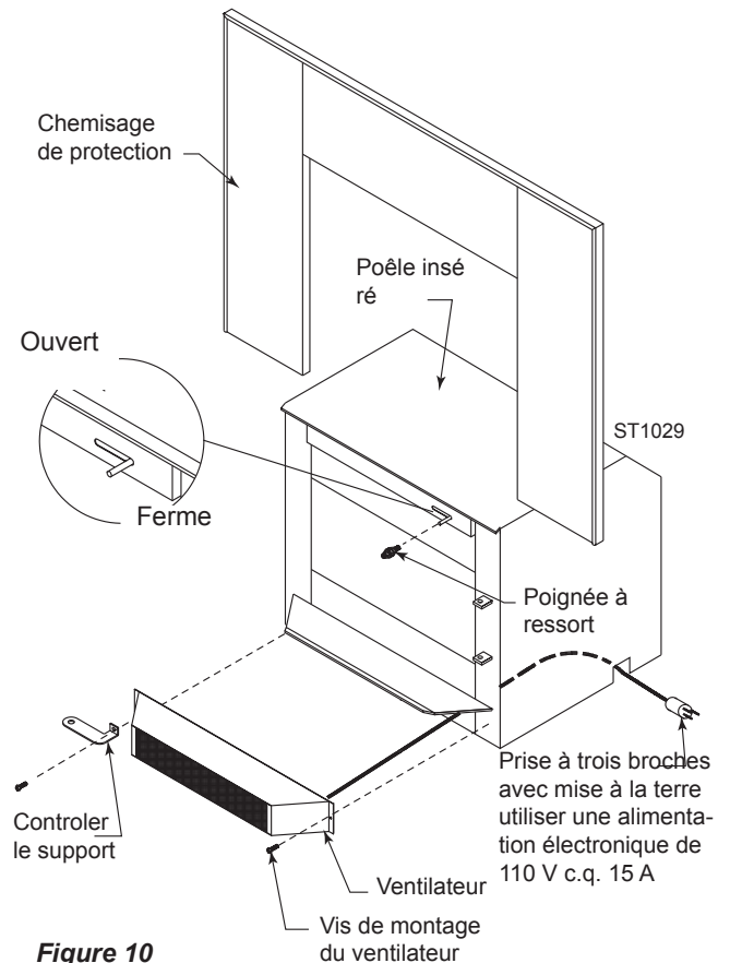
Figure 10 Installation du ventilateur
