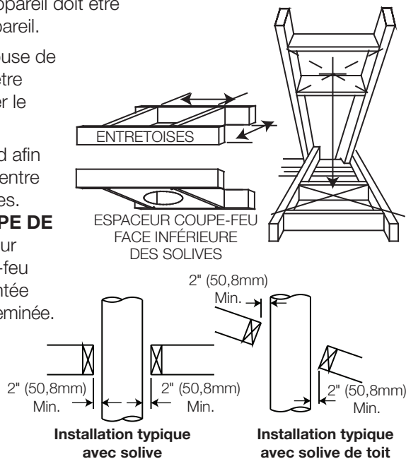
CHEMINÉE À DEUX DÉRIVATIONS
