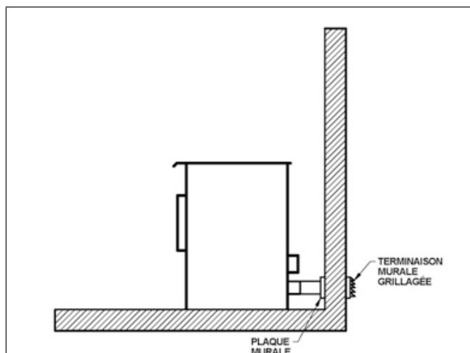
Prise d'air directement à l'extérieur
