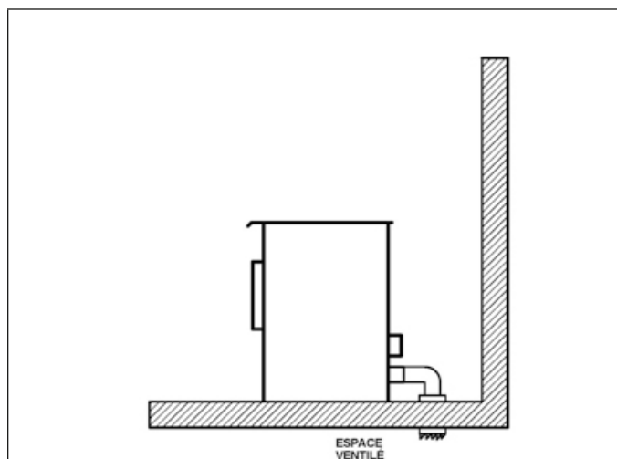
Prise d'air dans un espace ventilé
