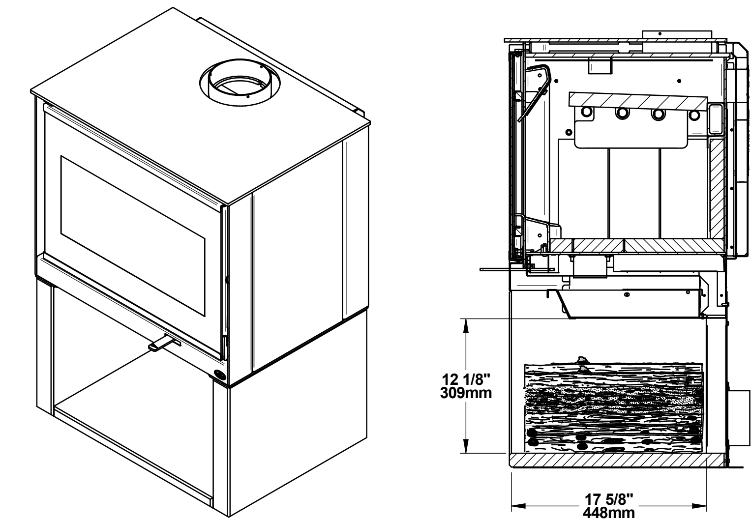
Base en pierre stéatite / Soapstone base
