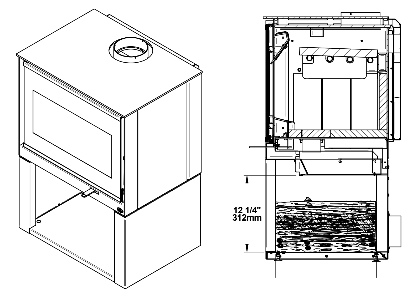
Base en acier / Steel base
